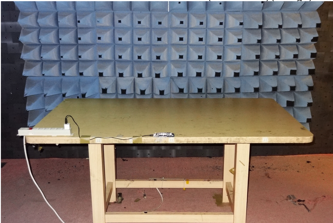
RADIATED ELECTROMAGNETIC FIELD (EN 61000-4-3) (Config 3)
